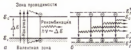
Рис. 1. Энергетические схемы: а — накачки и излучательной рекомбинации в полупроводнике; б — оптич. усиления при наличии инверсии населённости состояний вблизи краёв зон — дна \epsilon_c зоны проводимости и потолка \epsilon_v валентной зоны; \Delta \epsilon — ширина запрещённой зоны; \epsilon_f^e и \epsilon_f^d — квазиуровни Ферми для электронов проводимости и дырок.
